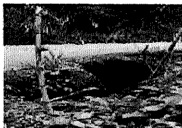
25 Fotos daño en alcantarilla camino San Juan Norte
